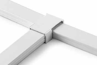
Ángulo "T" Troquele las paredes B y C "T" Angle Punch sides B and C
